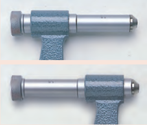
Применение с регулируемой опорой на детали
