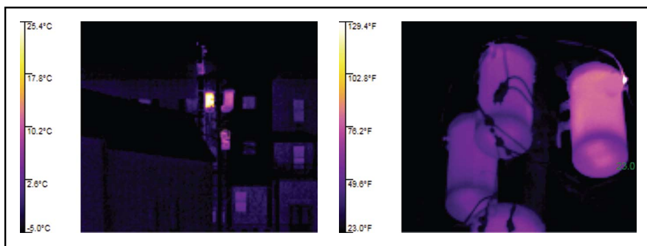
Рис. 5-35. Некоторые проблемы можно обнаружить даже на большом расстоянии (слева) с помощью тепловизора. Более тщательный анализ часто требует использования телескопического объектива или подойти ближе (справа) к оборудованию.
