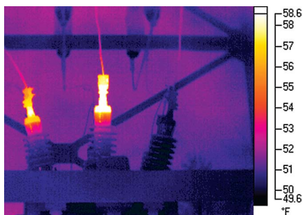
Рис. 5-59. Два из шести вводов маслонаполненного разъединителя имеют ненормальный нагрев и говорят о состоянии, которое может привести к серьезным финансовым последствиям, если бы его не выявили и не отремонтировали.
