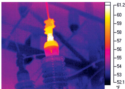
Рис. 5-55. Область в светлых цветах на маслонаполненном разъединителе говорит о том, что внутреннее соединение крышки ввода со стержнем является ненормально горячим.
