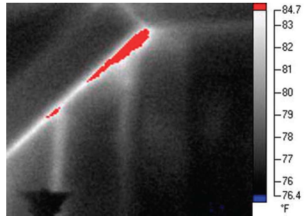
Рис. 5-43. Красный цвет насыщения цветовой палитры четко указывает плохую укладку теплоизоляции из стекловолна в наклонной кровле.
