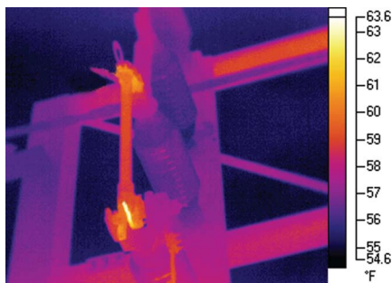
Рис. 5-34. Выявление таких проблем, как горячие губки и нож высоковольтного разъединителя, может быть несложным при условии адекватной нагрузки и небольшом ветре или его отсутствии.
