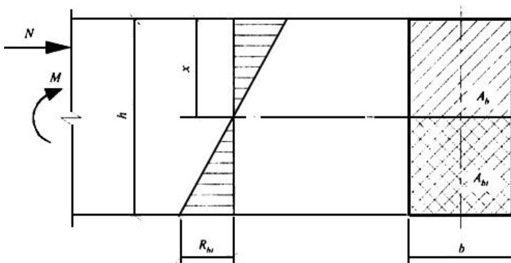
Рисунок 6.2 - Схема усилий и эпюра напряжений в сечении, нормальном к продольной оси изгибаемого (внецентренно сжатого) бетонного элемента, рассчитываемого по прочности с учетом сопротивления бетона растянутой зоны
