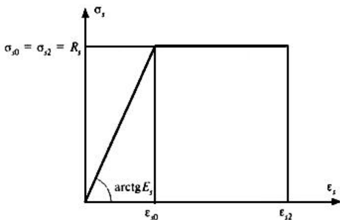
Рисунок 5.2 - Диаграмма состояния растянутой арматуры
