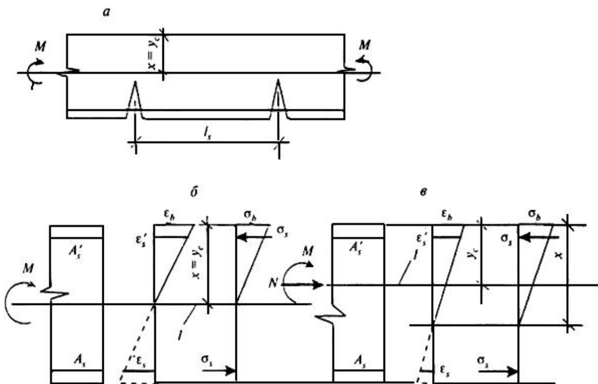
Рисунок 7.2 - Схема напряженно-деформированного состояния элемента с трещинами при действии изгибающего момента (а, б), изгибающего момента и продольной силы (в)
