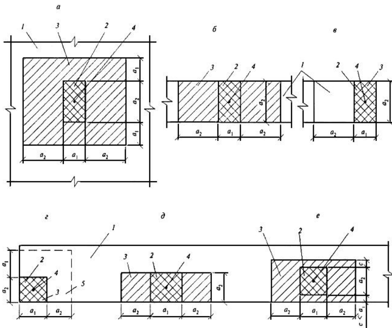
Рисунок 6.11 - Схемы для расчета элементов на местное сжатие при расположении местной нагрузки
