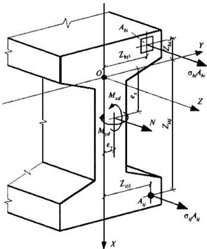
Рисунок 6.7 - Расчетная схема нормального сечения железобетонного элемента
