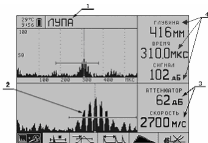
Рис. 3.6 Экран прибора в режиме ЛУПА (1 - название режима; 2 – отображение сигнала в стробе ; 3 - настройки прибора; 4 – измеряемые параметры сигнала)
