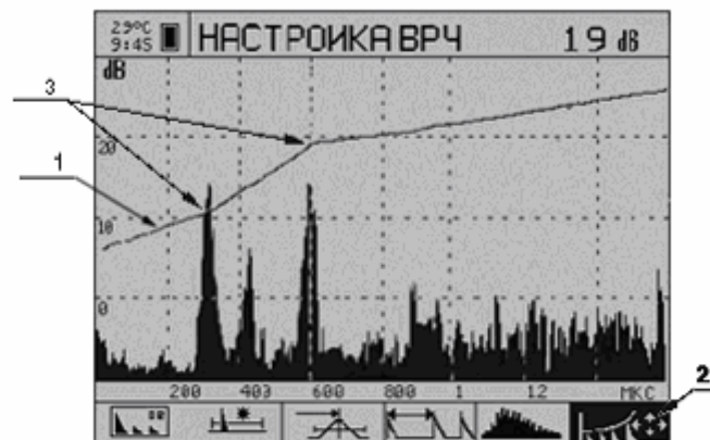
Рис. 3.5 Экран прибора при настройке ВРЧ. (1 – кривая ВРЧ ; 2 – активная пиктограмма ; 3 – узловые точки ВРЧ)
