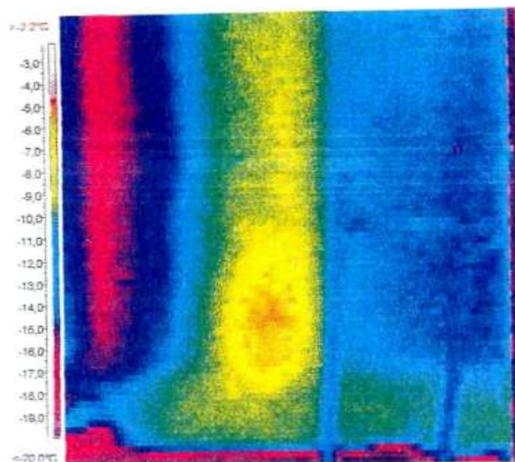
Рис. 1.7 Участок стены сооружения с повышенными теплопотерями. (Его границей следует считать изотерму -11^{\circ}\text{C} )
