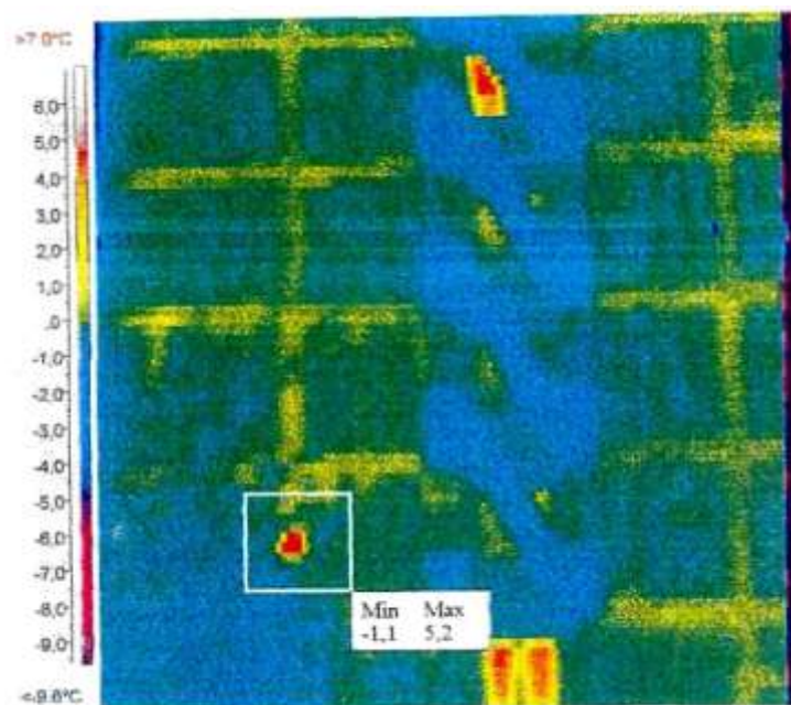
Рис.1.5 Термограмма стены панельного здания без оконных проемов. В левой части видно место воздухопроницания через межпанельный шов. (Соответствует температуре +5,2 °C)
