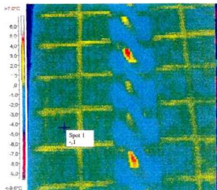
Рис.1.6 Термограмма стены панельного здания без оконных проемов. Участок с температурой -3 °C может быть принят как базовый
