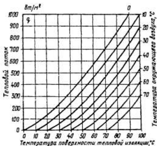
Номограмма для коэффициента излучения поверхности C = 2,67 Вт/(м·К)
