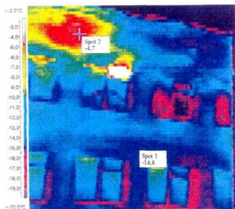
Рис.1.8 Термограмма малоэтажного кирпичного здания. В верхней части участок с повышенными теплопотерями. Фрагмент стены с температурой -14,8^{\circ}\text{C} здесь принят, как базовый
