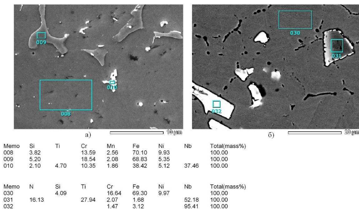
Рисунок 2 – Данные РСМА в различных областях исходного образца а) в металле шва и б) в основном металле.
