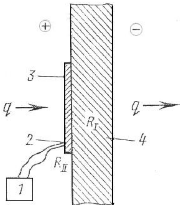
Рисунок 1 - Схема измерения плотности теплового потока
