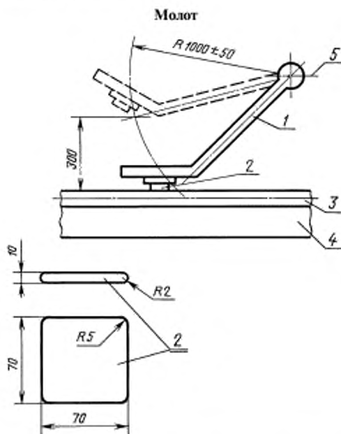
1 — молот; 2 — лопка; 3 — ампульпровод; 4 — горизонтальная плита массой 150 кг; 5 — горизонтальная ось
