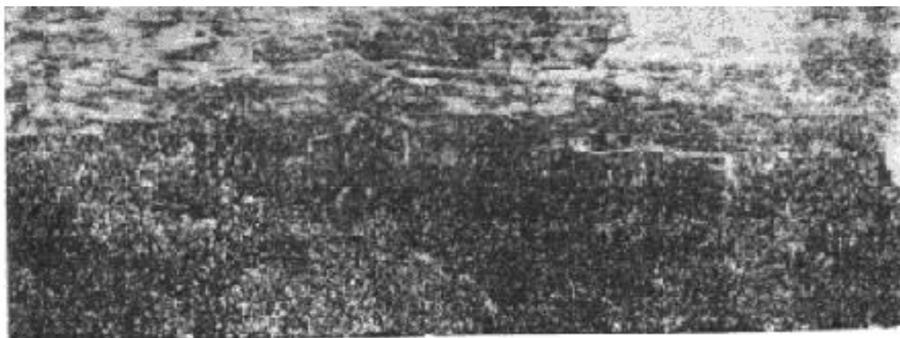
Рис. 61. Шлифовочные трещины
