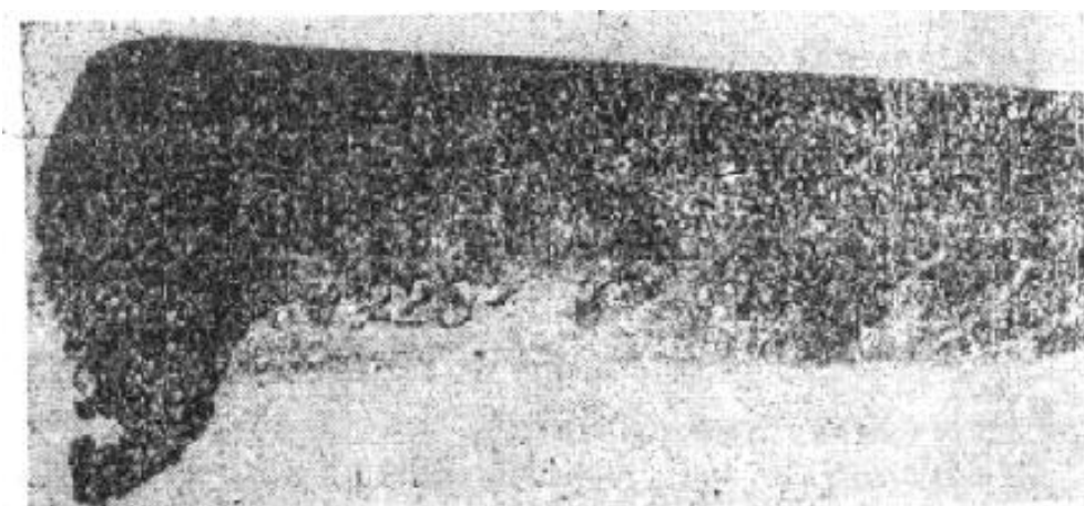
Рис. 54. Травильные трещины
