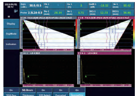
Моделирование сварного шва
