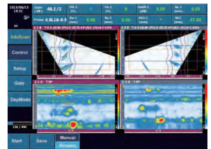
Две пары В+D развертки
