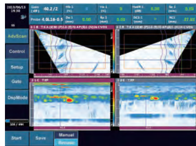
Две пары В+С развертки
