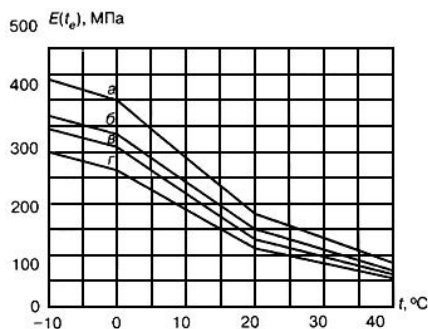
Рисунок 3 - Значения модуля ползучести \sigma материала труб для проектируемого срока эксплуатации 50 лет в зависимости от температуры транспортируемого газа
