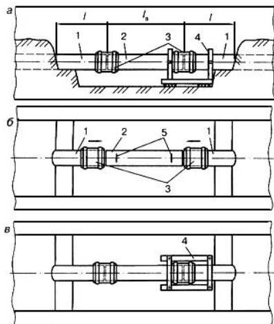
Рисунок 17 - Схемы освобождения газопровода в траншее от грунтовой присыпки (а) и последовательности вварки трубной вставки с применением муфт с закладными нагревателями (б, в)
