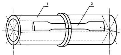
1 - патрубок со сварным соединением; 2 - расположение образцов
