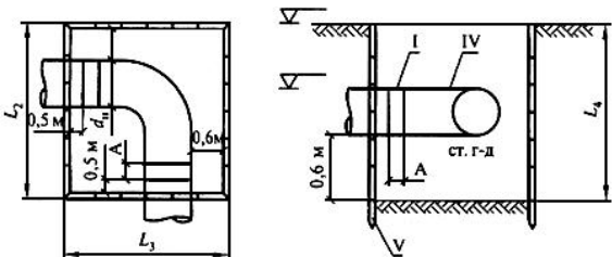
Рисунок Л.3 - Вставка отвода
