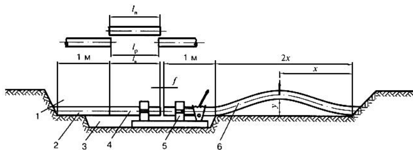
Рисунок 16 - Схема освобождения газопровода от грунтовой присыпки по длине и вварки трубной вставки встык
