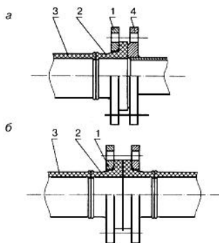
Рисунок 15 - Фланцевые соединения
