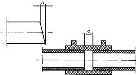
Рисунок 13. Величина косого среза торца трубы
