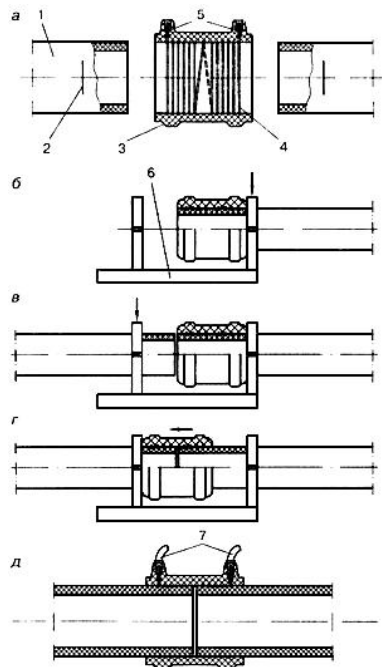
Рисунок 12 - Схема соединения труб муфтой с закладным нагревателем
