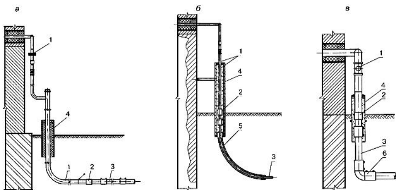
Рисунок 1 - Цокольные вводы газопровода в здание
