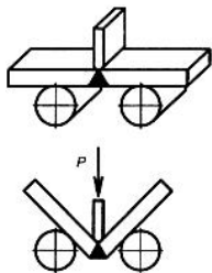
Рисунок Ф.1 - Схема испытания на статический изгиб
