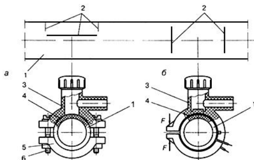
Рисунок 14 - Соединение полиэтиленовой трубы и отводов с закладными нагревателями
