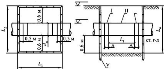
Рисунок Л.1 - Вставка стальной катушки
