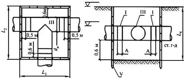
Рисунок Л.2 - Вставка тройника
