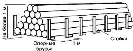
Рисунок 9 - Хранение отдельных труб в штабеле
