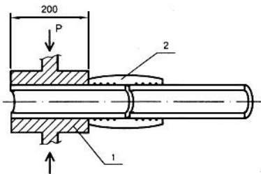
1 - обжимные плиты; 2 - испытываемый образец
