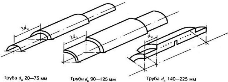
Рисунок Т.1 - Общий вид образцов-сегментов
