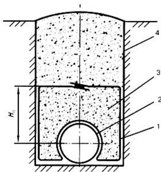
Рисунок Г.1 - Схема балластировки газопровода
